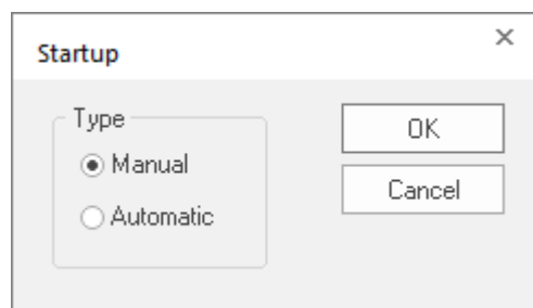
Startup
